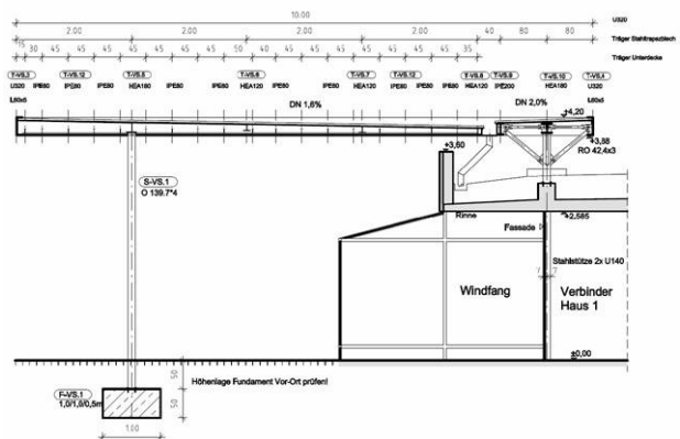
Vordach Süd, Berechnung Tragwerk
