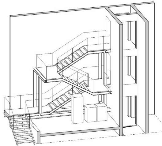
3D-Modell Berechnung Stahlterasse 2
